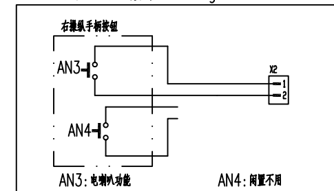
右操纵手柄电气接线图 Right Control
