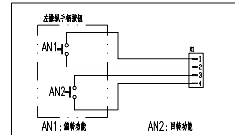
左操纵手柄电气接线图 Left Control
